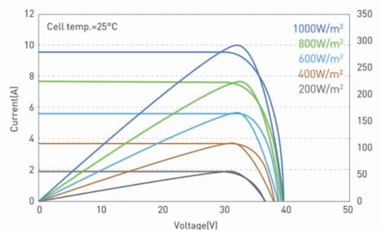
不同辐照度下电流电压曲线 / 功率电压曲线 (290W)
