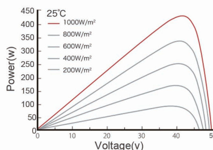
Power-voltage(420W)
