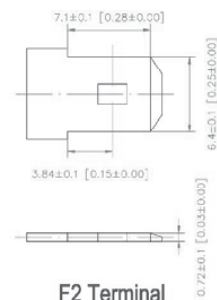
F2 Terminal
