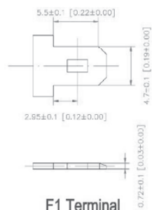
F1 Terminal
