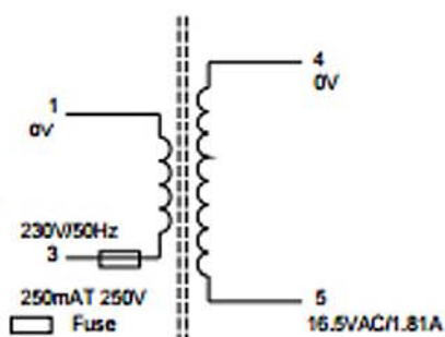
SCHEMATIC(电路原理图):
